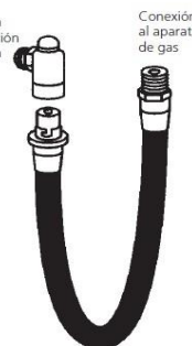
Tubo flexible espirometálico con enchufe de seguridad
